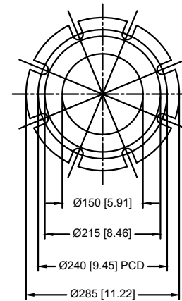
DISCHARGE FLANGE 3" 150LB ANSI RF
