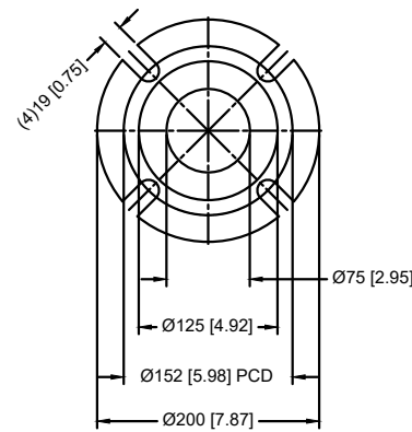
DISCHARGE FLANGE 3" 150LB ANSI RF
